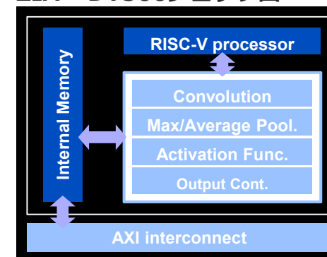
ZIA™ DV500ブロック図
